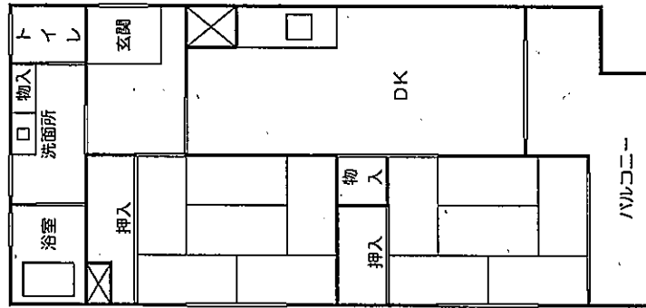
形式：2DK 箱塚団地 中耐4階建
